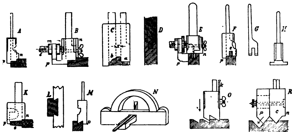
Č. 1727. Hoblíky truhlářské.
